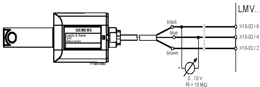
Рис. 17 - Детектирование с фотоэлементом QRI..
