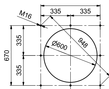
Рекомендуемая амбразура котла
