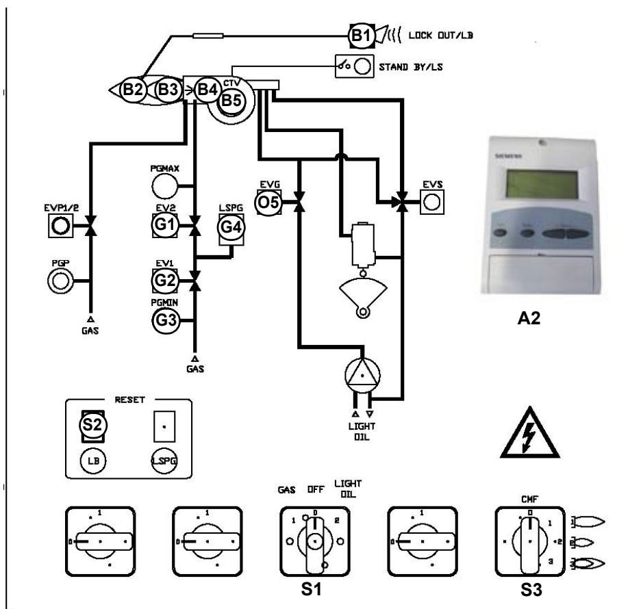
Рис. 8 - Лицевая панель электроцита
