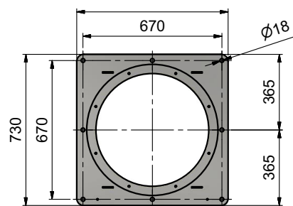
Фланец горелки
