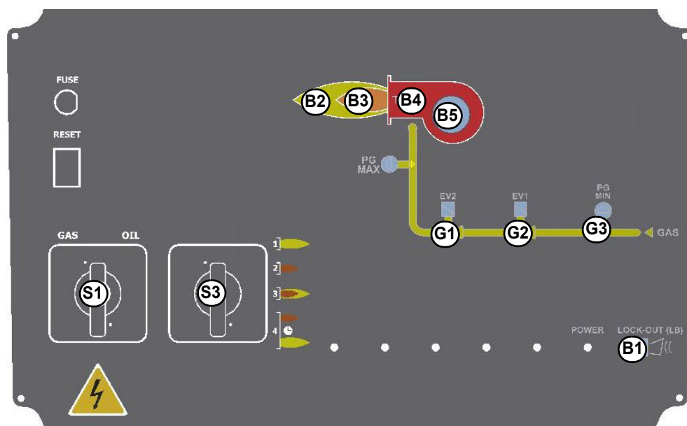
Рис. 5: передняя панель электрощита горелки
