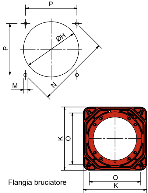
Foratura caldaia consigliata
