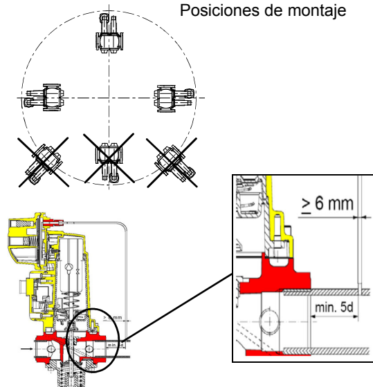
SIEMENS VGD.. Posiciones de montaje
