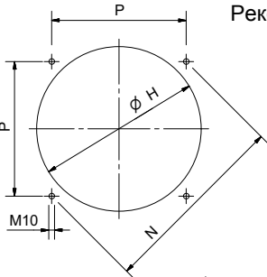
Фланец горелки
