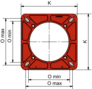
Фланец горелки
