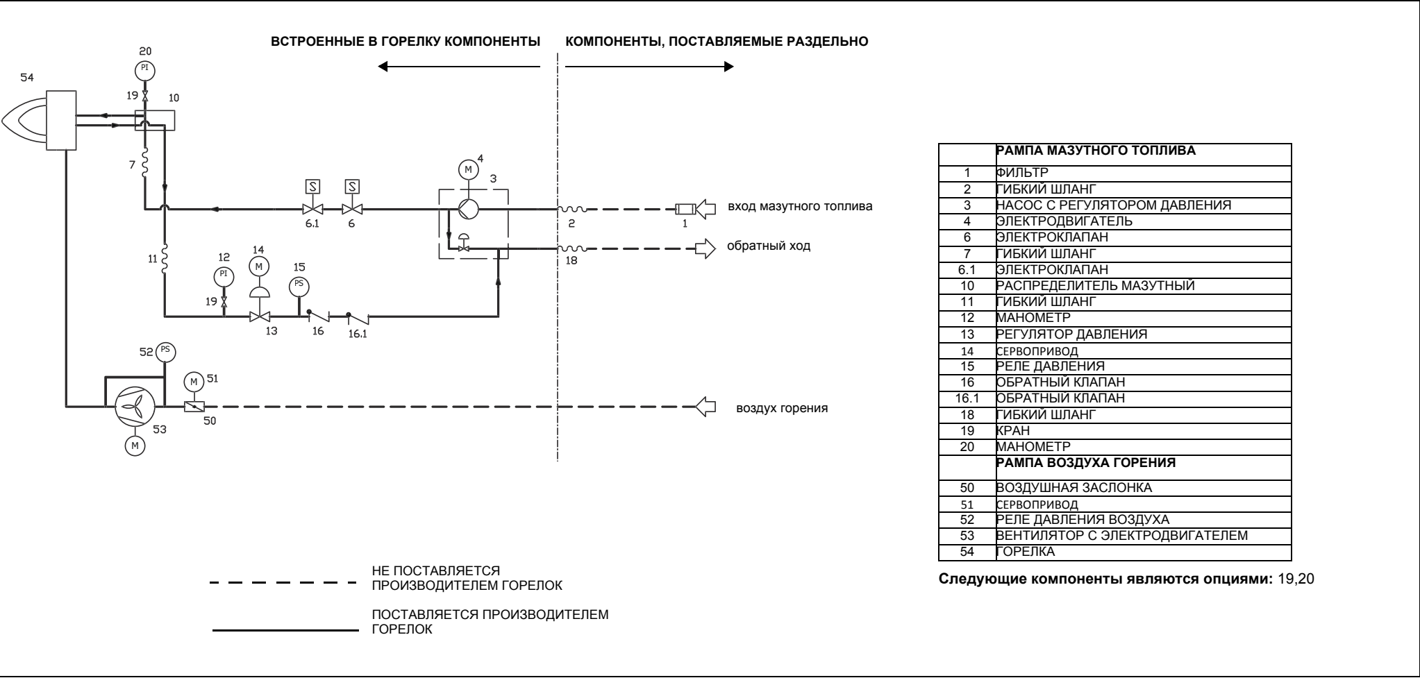
Рис. 4 - 3/2G23 v0 – Гидравлическая схема
