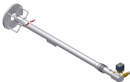
Рис. 13 - Голова сгорания с фурмой дизтоплива (PG70 - PG81)
