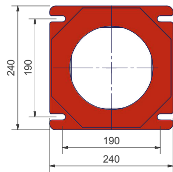
Фланец горелки
