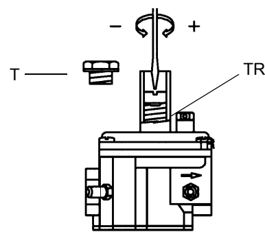
Стабилизатор давления
