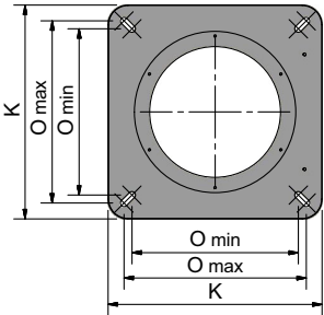
Plantilla de perforación de la placa
