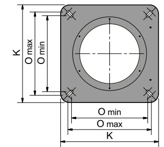
Фланец горелки
