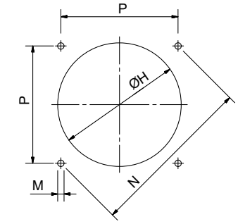
Схема сверления плиты котла
