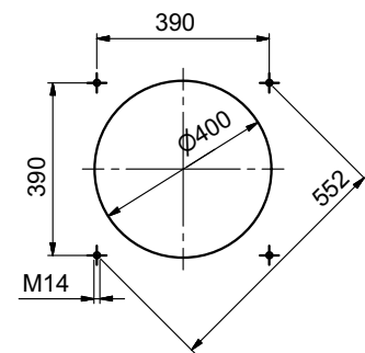
Plantilla de perforación
