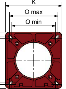
Фланец горелки
