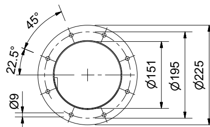
фланец FGR
