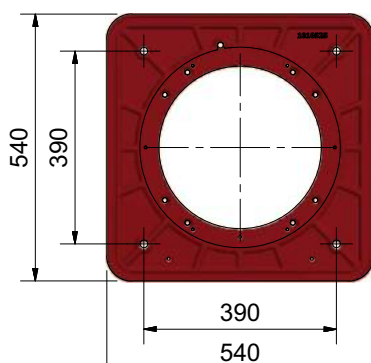
Фланец горелки
