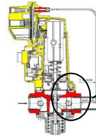
Siemens VGD... с SKPx Пример газовой рампы
