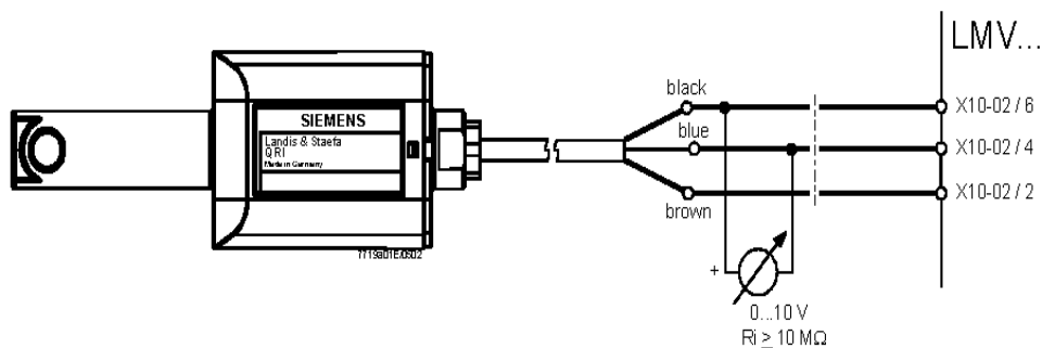
Рис. 11 - Детектирование с фотозлементом QRI..
