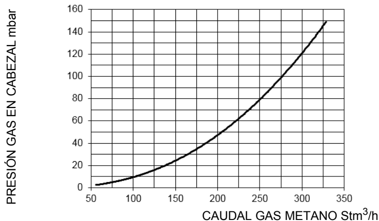
N1060X L-..
