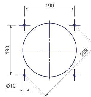
Foratura caldaia
