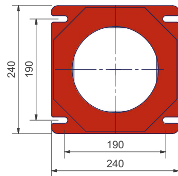
Flangia bruciatore
