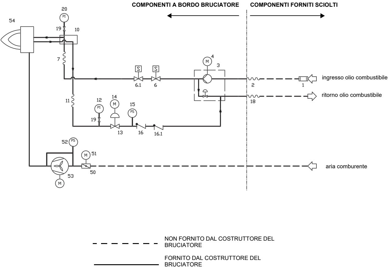
Fig. 5 - 3I2G-23 v0 Schema idraulico
