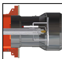
posizione "MAX"
