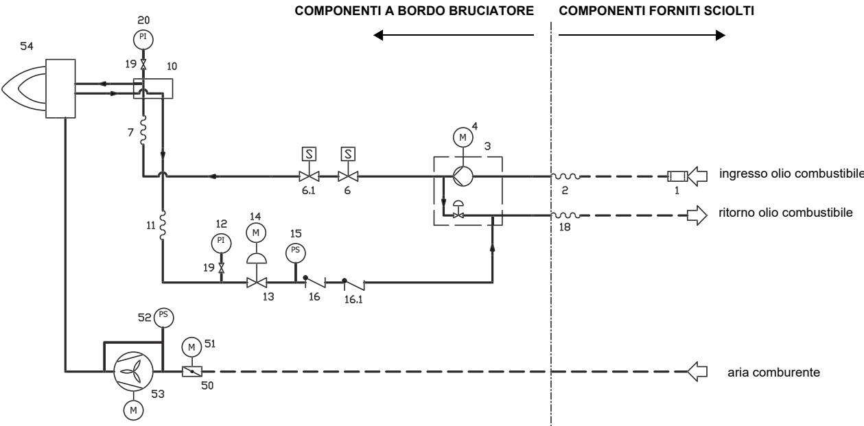
Fig. 5 - 3I2G-23 v0 Schema idraulico
