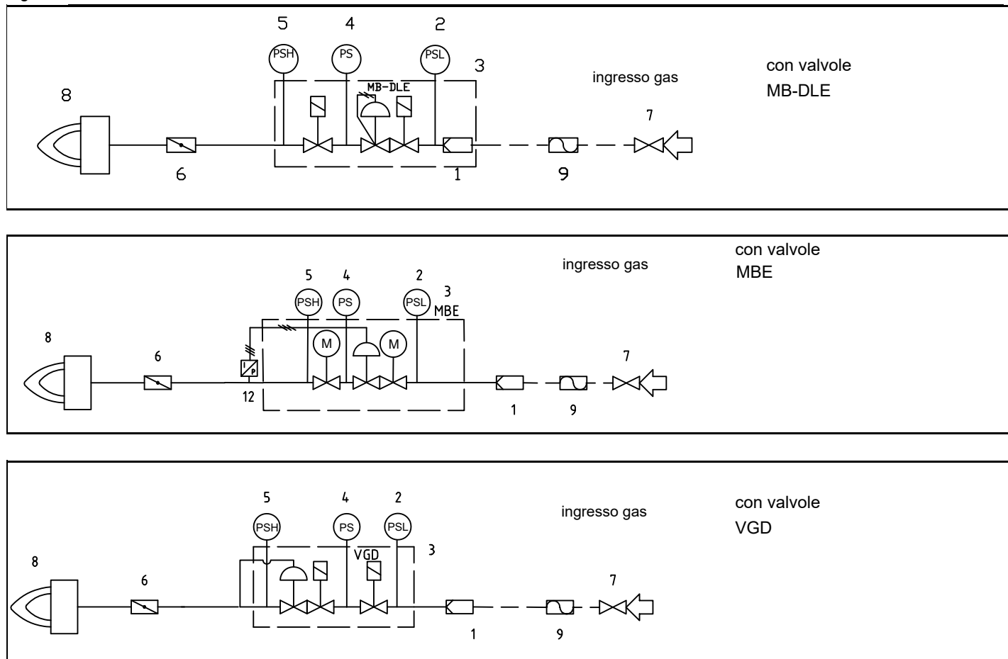
Fig. 5 - - Schema idraulico
