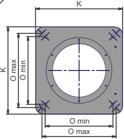
Flangia bruciatore
