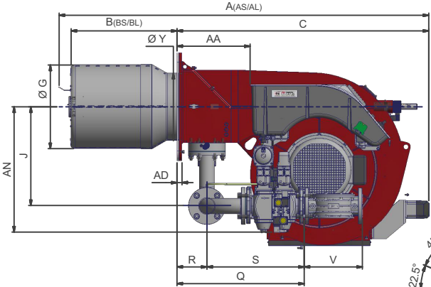
FLANGIA FGR
