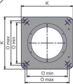
Brida quemador
