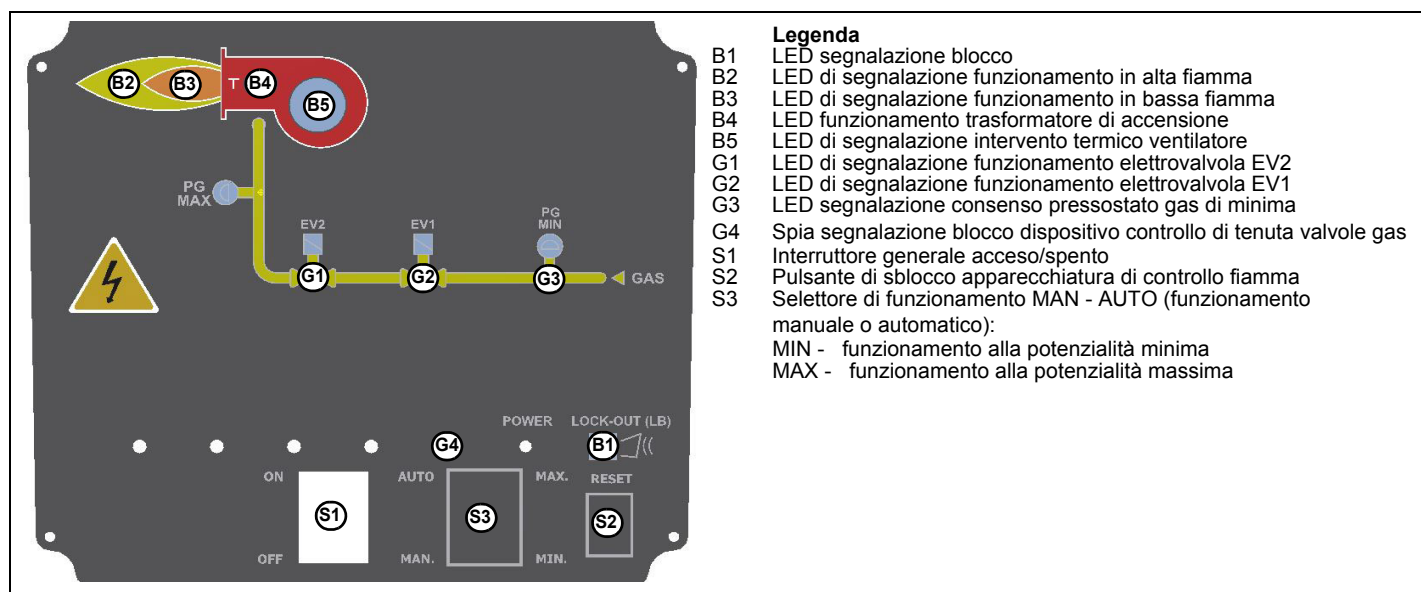
Fig. 4 - Pannello frontale quadro elettrico bruciatore
