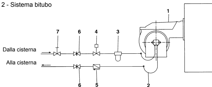
Fig. 2 - Sistema bitubo
