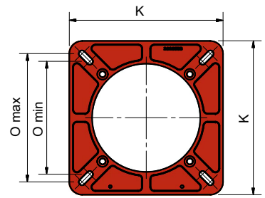
flangia bruciatore
