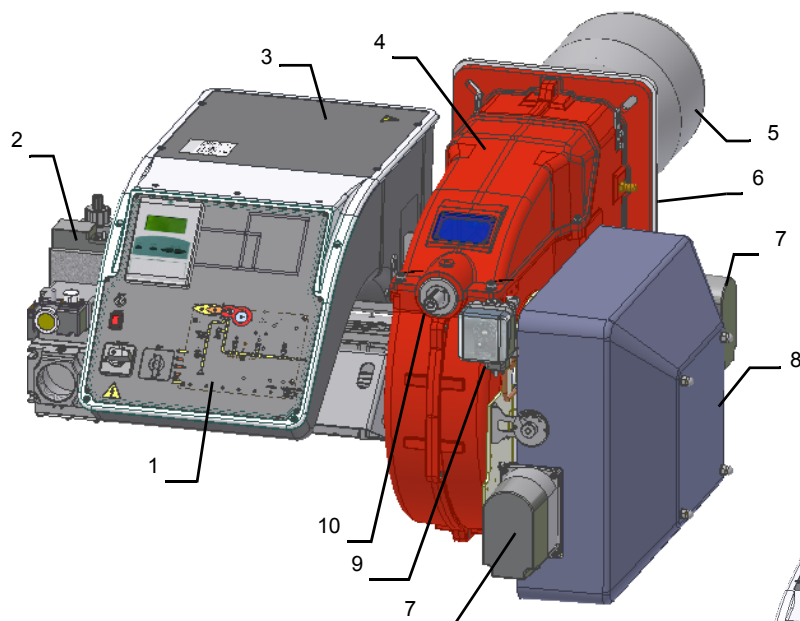
Bruciatore con cassetto aspirazione aria in polimero ABS (silenziato)
