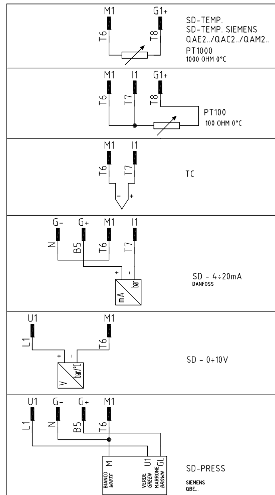
Fig. 21 - Raccordement sondes
