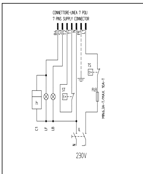
Fig. 19 - Brûleurs modulants
