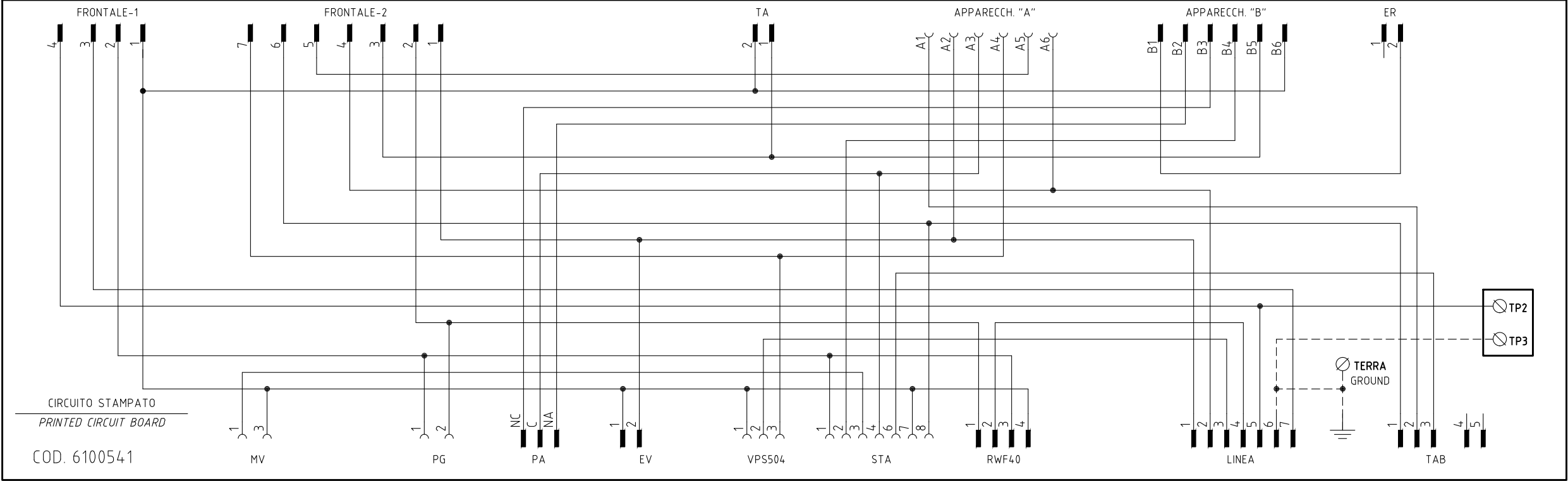
FRONTALE-1
