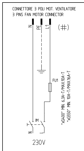
Fig. 16 Branchement moteur électrique NG/LG/NGX400
