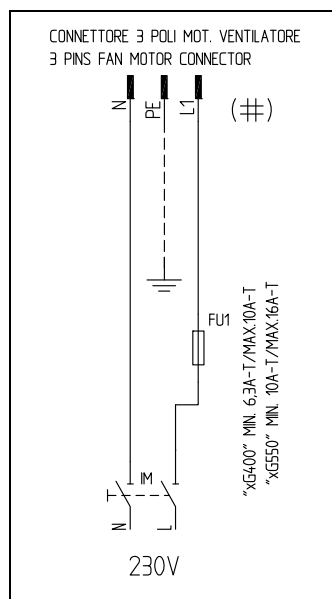
Fig. 18 Branchement moteur électrique NG/LG/NGX400
