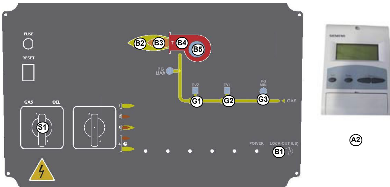
Рис. 4: передняя панель электрощита горелки
