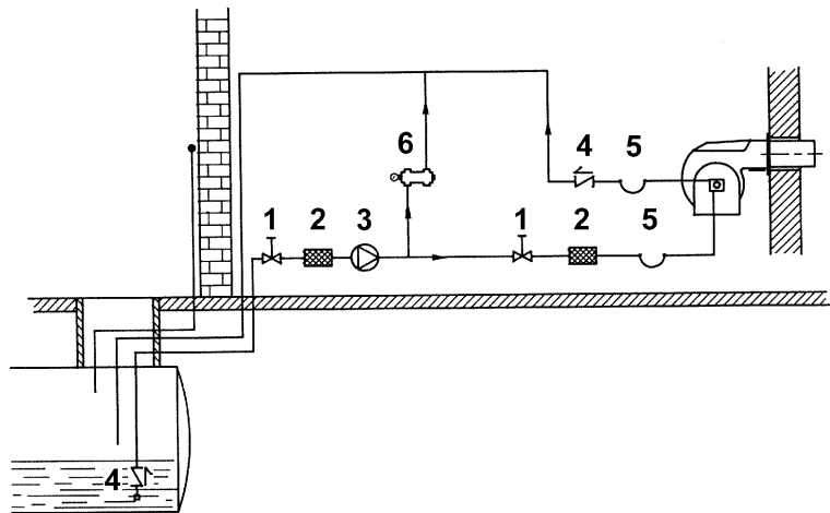
Рис. 8 - Кольцевой контур подачи топлива
