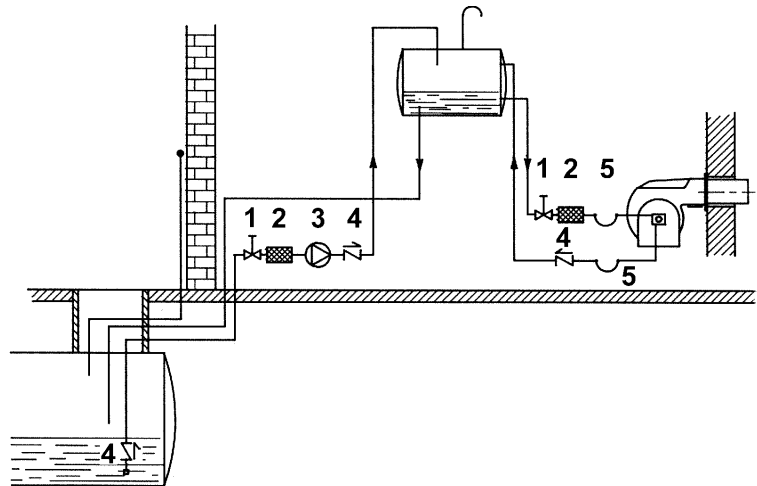
Рис. 7 - Контур подачи топлива под силой гравитации
