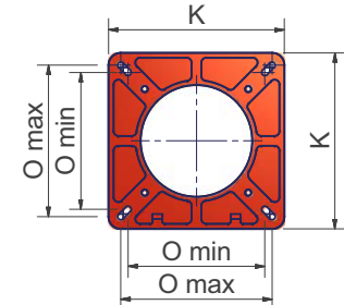
Фланец горелки
