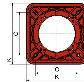
Фланец горелки
