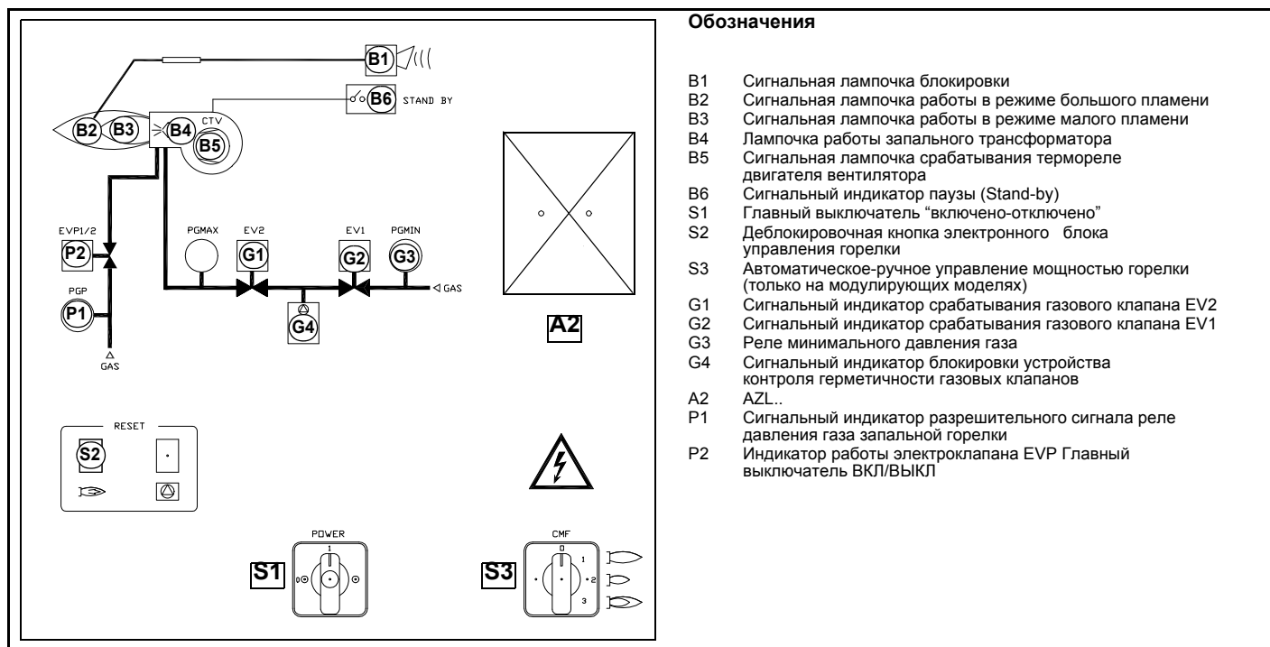
Рис. 5 - Лицевая панель электрощита
