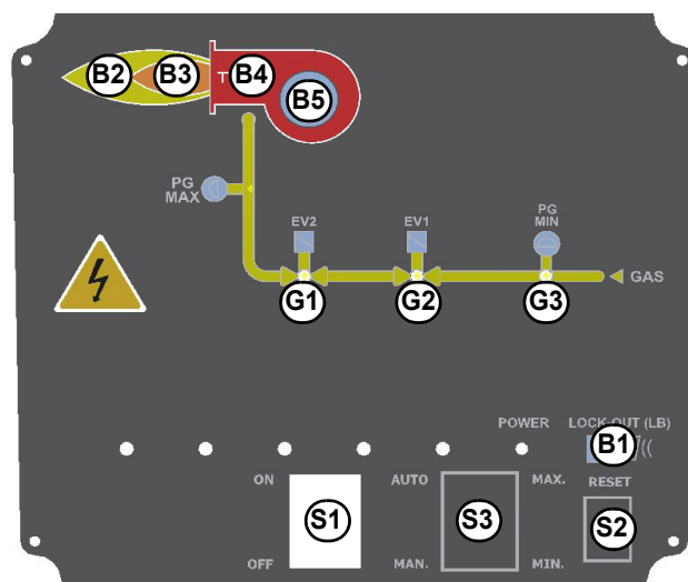
Fig. 1 - Pannello frontale quadro elettrico bruciatore
