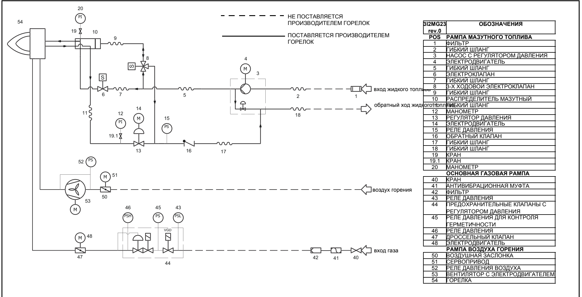
Рис. 4 - 3I2MG23 v0 – Гидравлическая схема
