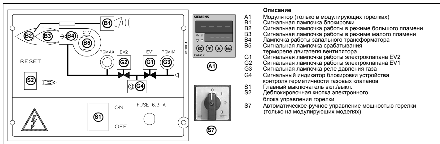
Рис. 13: передняя панель электрощита горелки
