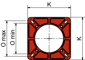
Фланец горелки
