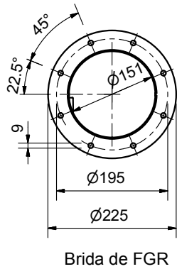
Brida de FGR
