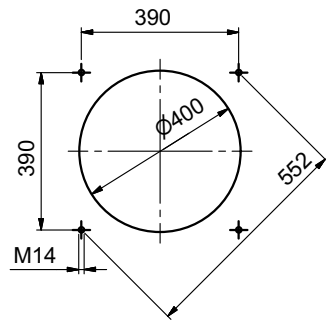
Plantilla de perforación
