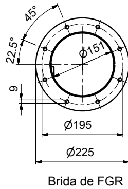
Brida de FGR
