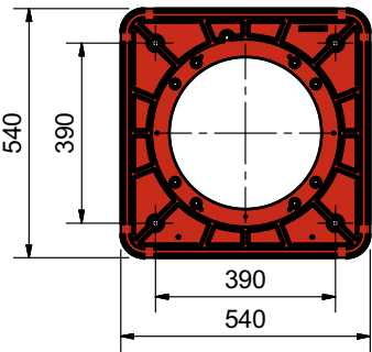
brida de quemador.
