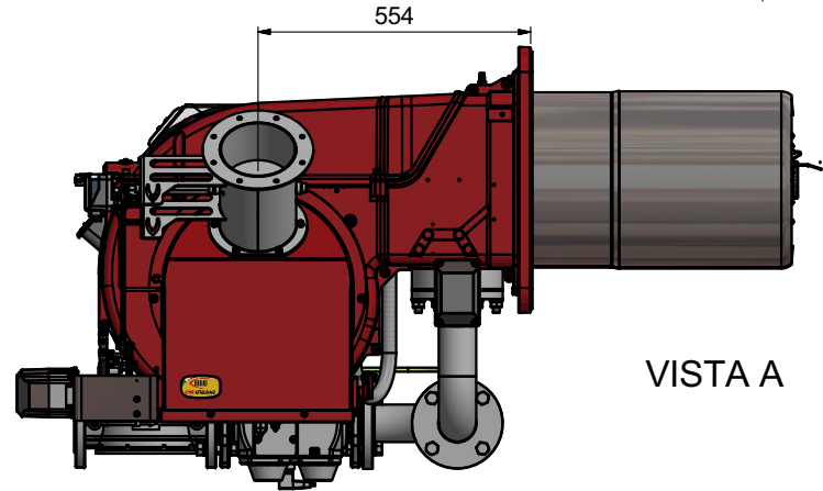
Brida de FGR
