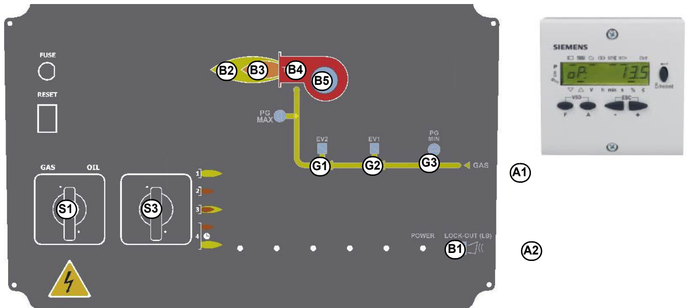
Fig. 6 Panel frontal cuadro eléctrico
