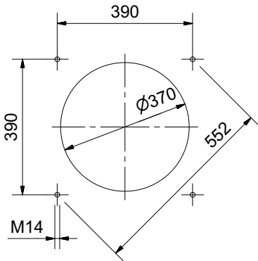
Plantilla de perforación
