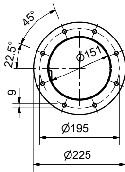
Brida de FGR
