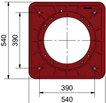
brida de quemador.
