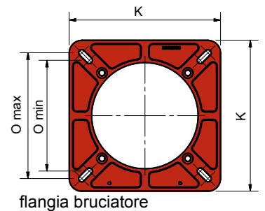
flangia bruciatore
