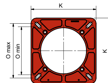
flangia bruciatore
