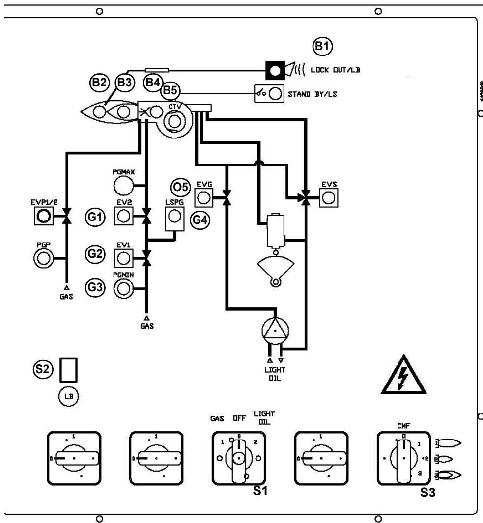
Рис. 6 - Лицевая панель электроцита
