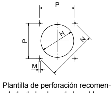
brida de quemador.
