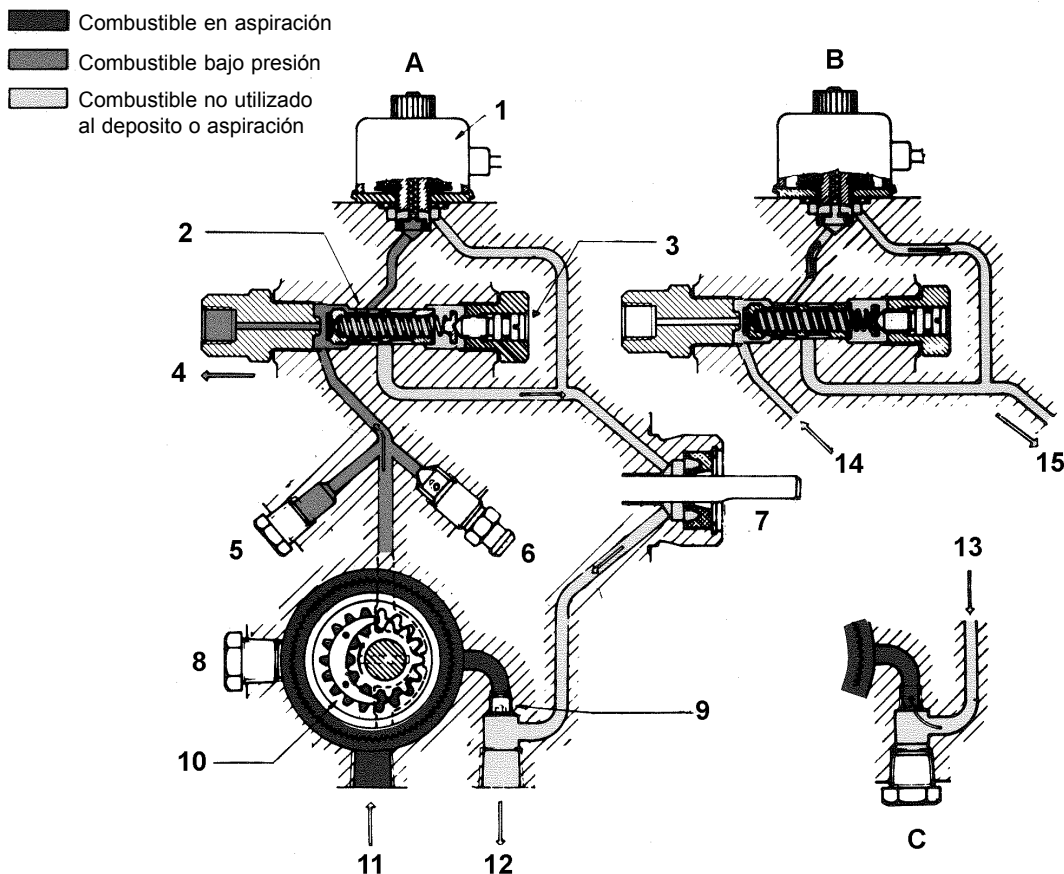
INSTALACIÓN A 2 TUBOS
