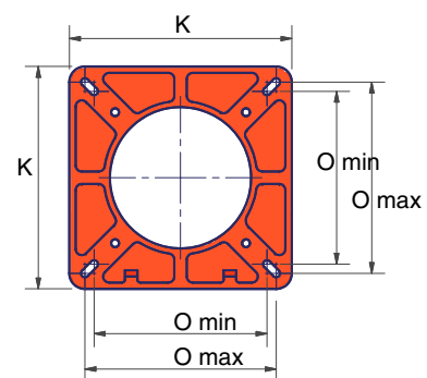
Фланец горелки
