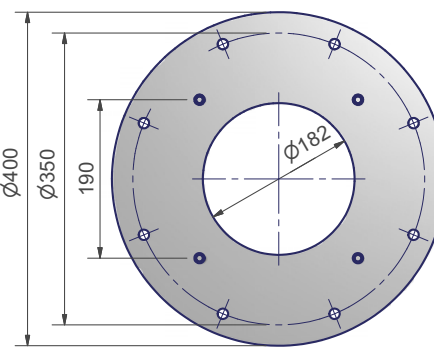
Рекомендуемый контрфланец
