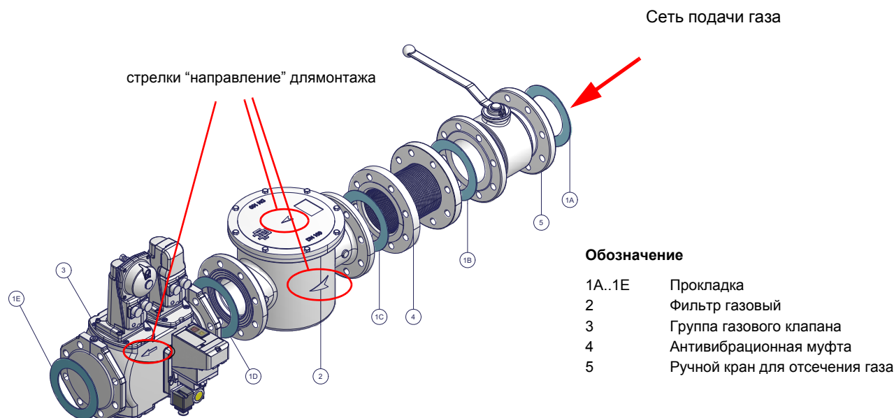
Рис. 3 - Пример газовой рампы
