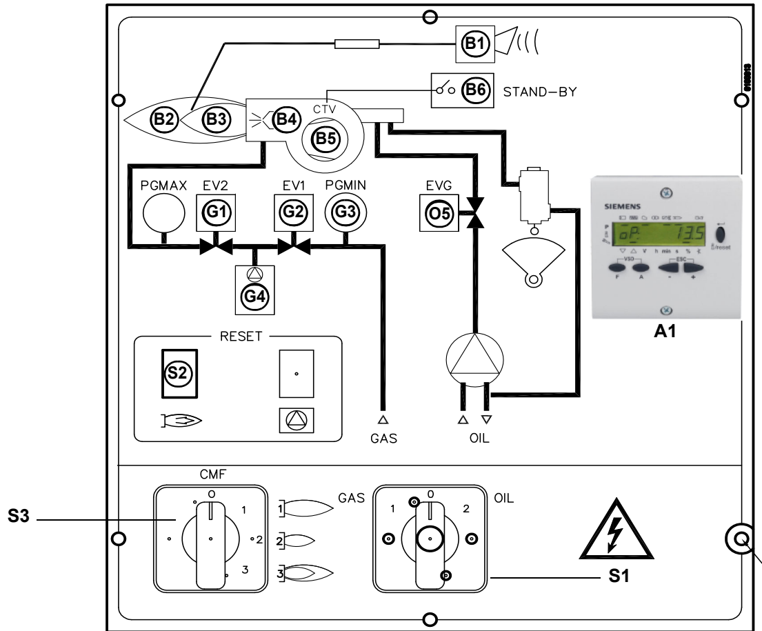
Fig. 4 - Panelo cuadro electrico
