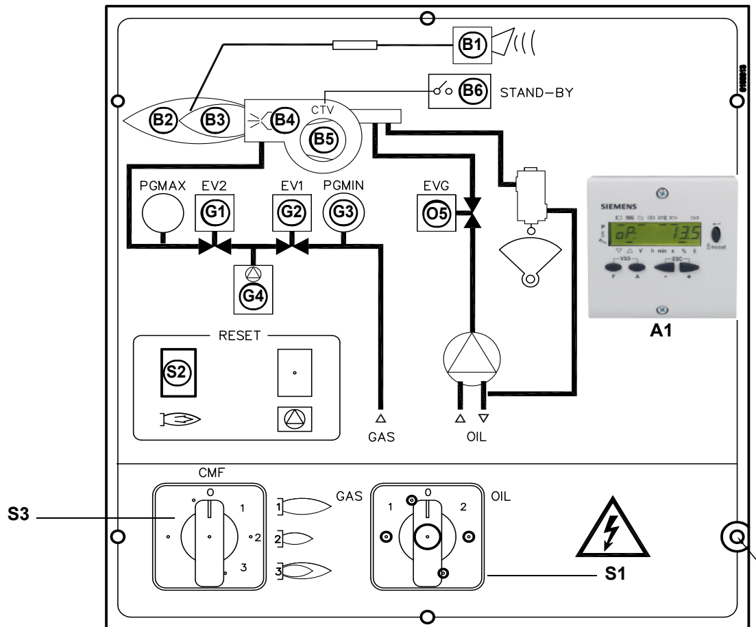
Fig. 4 - Pannelo cuadro electrico
