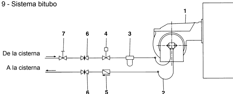
Fig. 9 - Sistema bitubo
