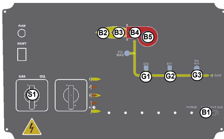
Fig. 3 - Pannello frontale quadro elettrico bruciatore
