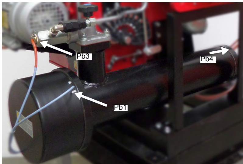
Рис. 19 Подключение датчиков DANFOSS MCX
