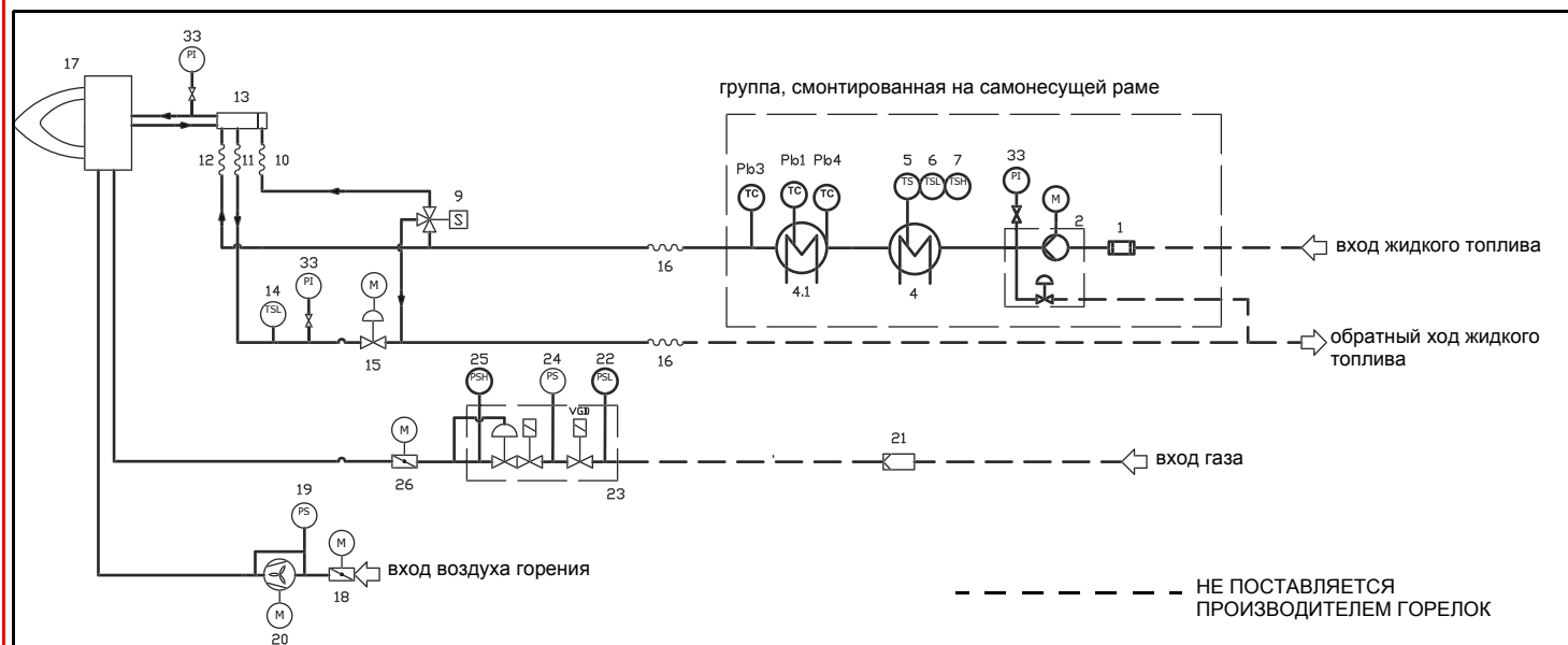
Рис. 5 Гидравлическая схема 3I2MG23 v0
