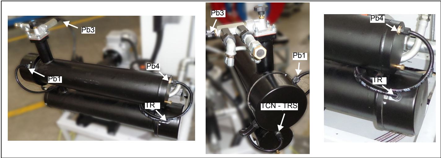
Рис. 20 (Горелки с двойным бачком - подогревателем)Подключение датчиков DANFOSS MCX и подключение термостатов
