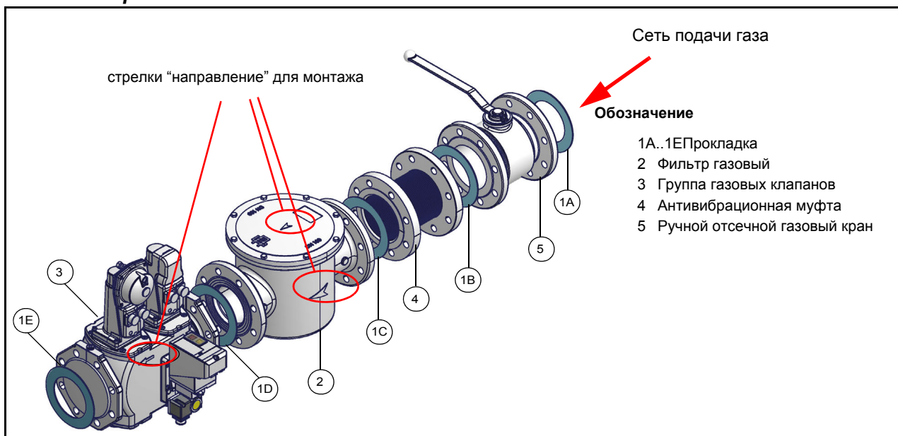
Рис. 6 - Пример газовой рампы Fig. 7
