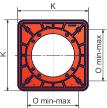
Рекомендуемый фланец горелки
