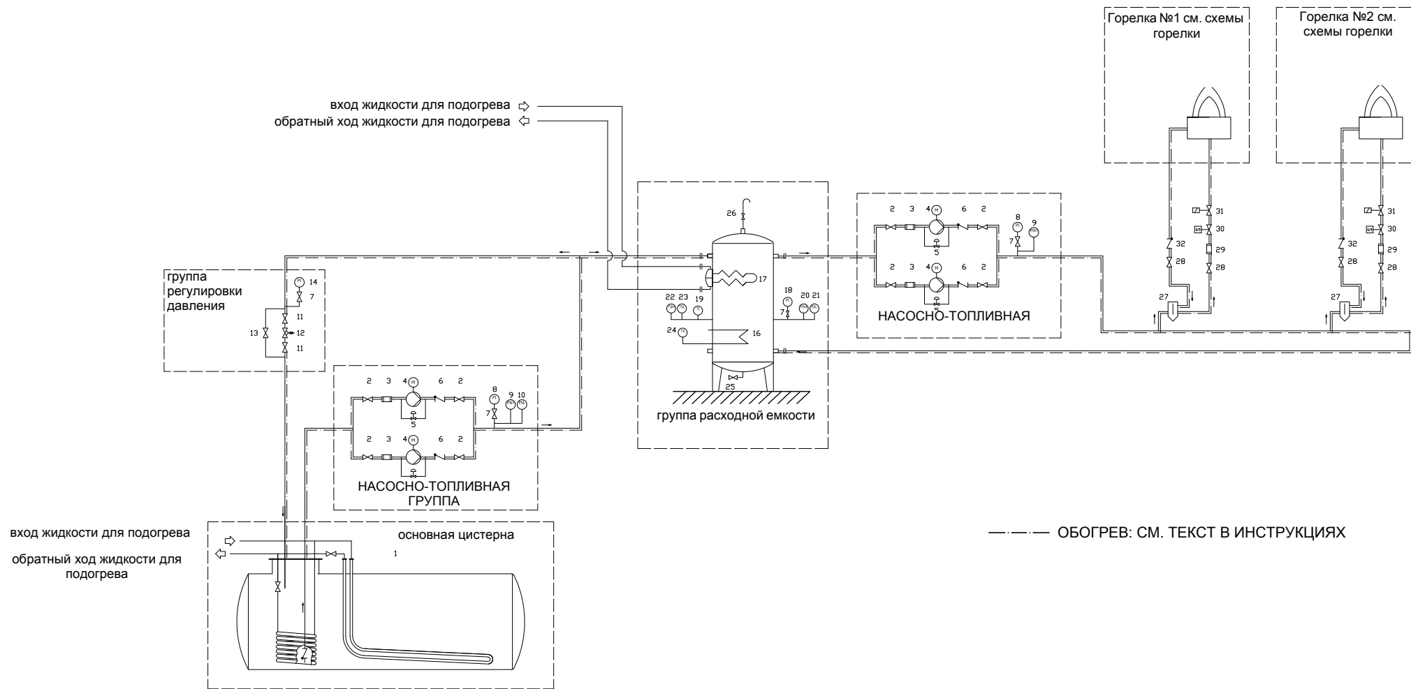
Рис. 15 Гидравлическая схема 3ID0014 v2- Система подачи мазута при наличии от двух и более горелок
