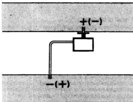
С – Измерение разницы давления между двумя каналами
