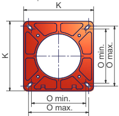
Рекомендуемый фланец горелки
