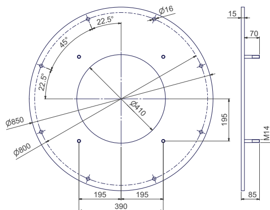
Рекомендуемый контрфланец
