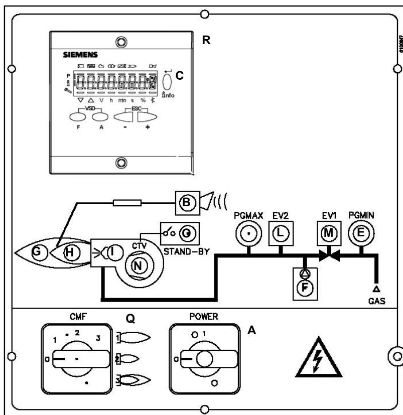
Fig. 6 - Panel de control del quemador
