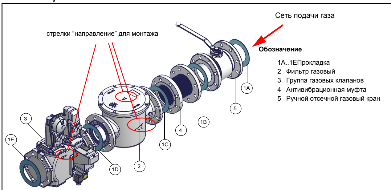
Рис. 6 - Пример газовой ramпы Fig. 7
