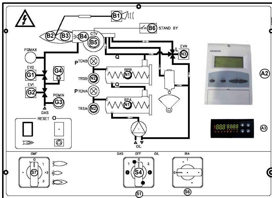
Рис. 21: передняя панель электроцита горелки
